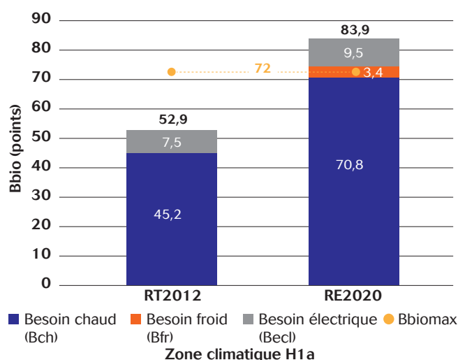
Fig. 1 Exemple d'évolution du Bbio entre la RT2012 et la RE2020 (pour un bâtiment type et à prestation égale)
